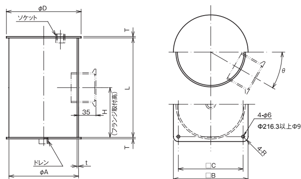
寸法図
